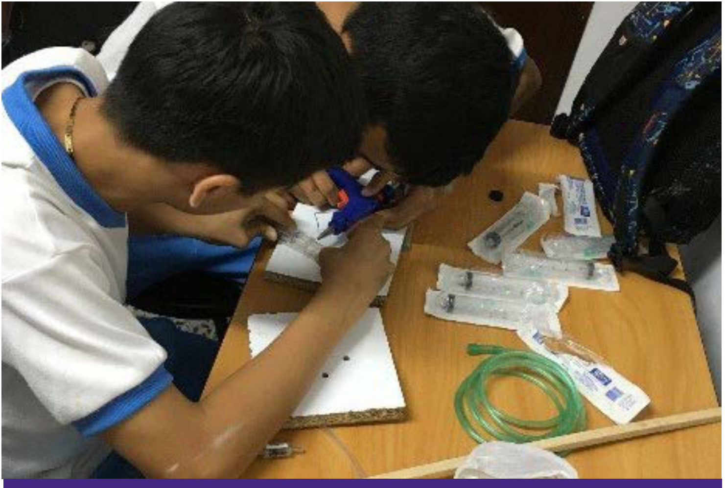
Experimento de Física: construcción prensa hidráulica. Fuente propia
